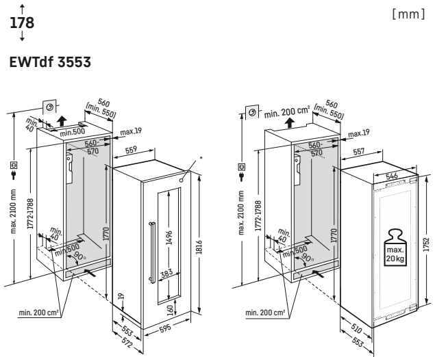
* Na zdjęciach widoczna rama ze stali szlachetnej. Wymiary drzwi w mm (sz/ wys/ gł): 595/1816/19 mm.
