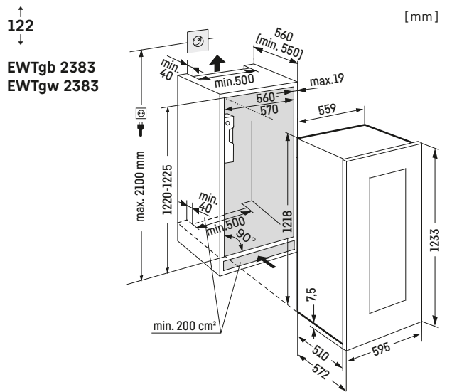
Wymiary drzwi w mm (sz/ wys/ gł): 595/1233/19 mm.
