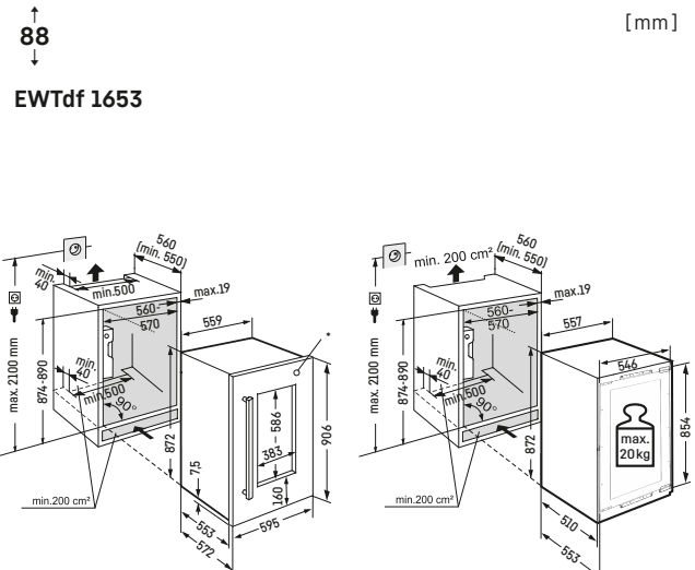
* Na zdjęciach widoczna rama ze stali szlachetnej. Wymiary drzwi w mm (sz/ wys/ gł): 595/906/19 mm.
