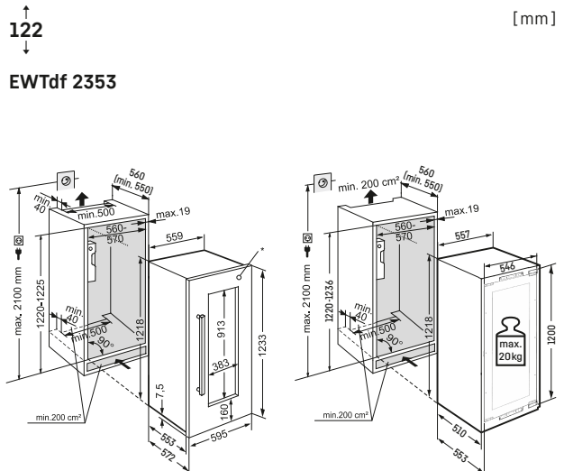
* Na zdjęciach widoczna rama ze stali szlachetnej. Wymiary drzwi w mm (sz/ wys/ gł): 595/1233/19 mm.
