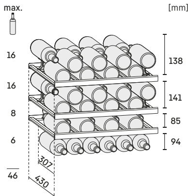
Schemat przechowywania: UWKes 1752 UWTes 1672
